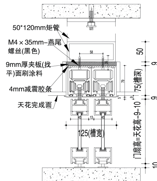
XP-A系列 窄盖双轨单开/双开门 双轨反向同步门
