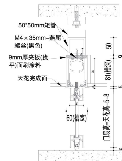
QM系列-40暗装 单轨单开门 单轨反向同步门 单轨口袋门
