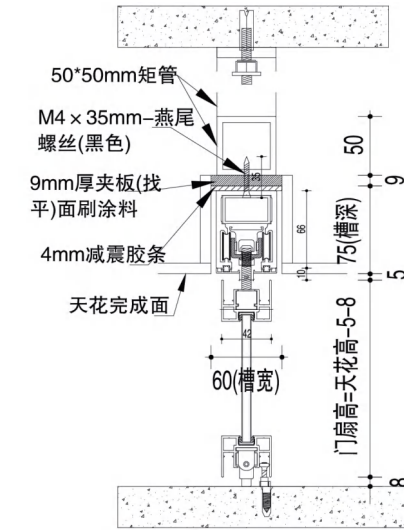
WP-B系列 窄盖单轨单开门 单轨反向同步门 单轨口袋门
