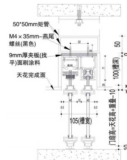
QM系列-40明装 双轨2+0联动门
