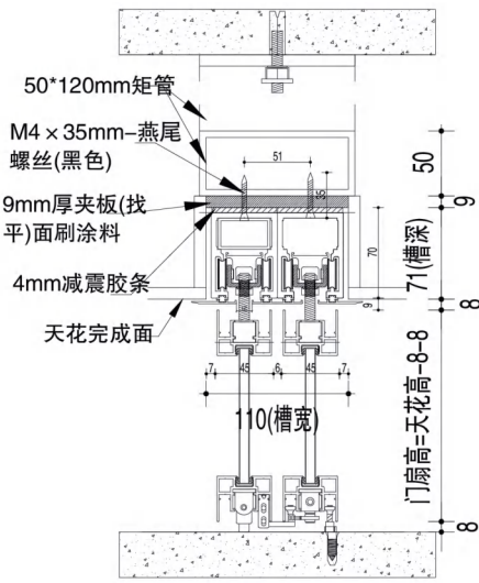
WP-A系列 宽盖单轨单开门/双开门 双轨反向同步门 双轨2+0联动门
