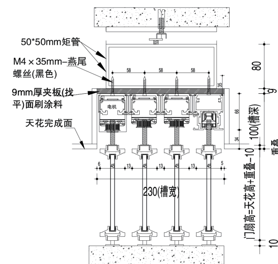
QM系列-45明装 三轨3+1联动门
