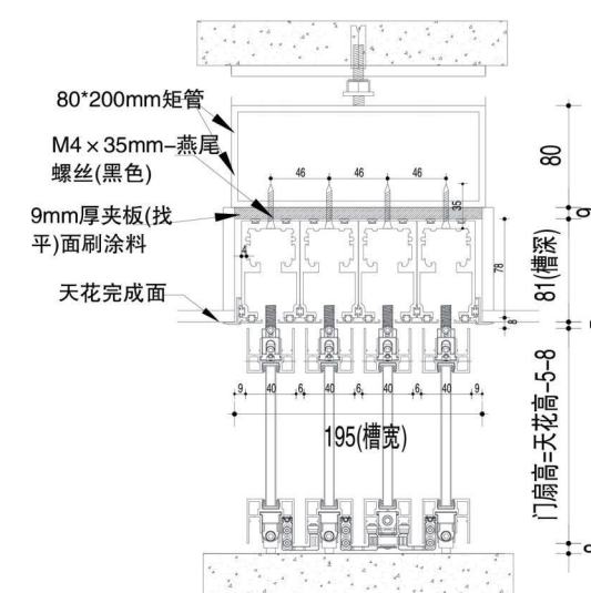
QM系列-40暗装 四轨3+1联动门
