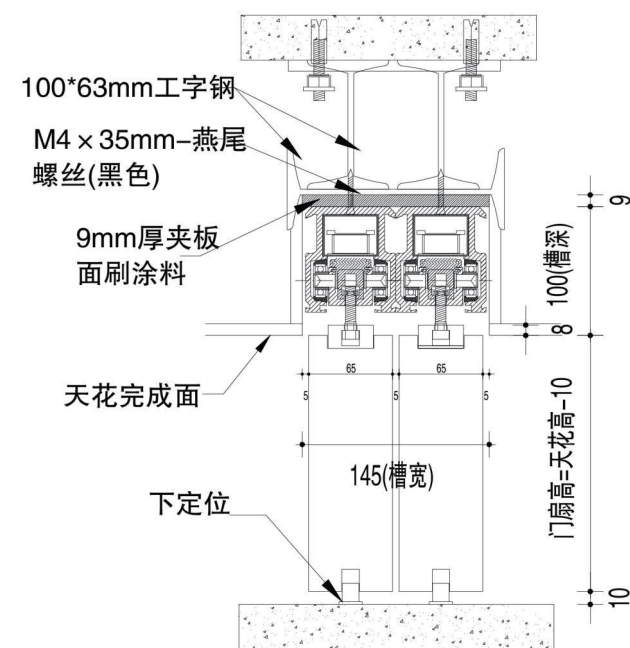
重型系列 双轨单开移门 双轨反向同步移门
