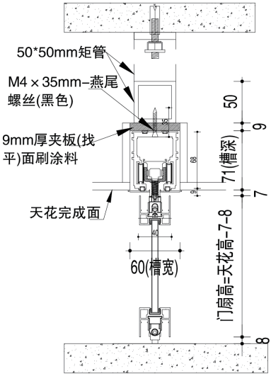
WM-A系列 宽盖单轨单开门 单轨反向同步门 单轨口袋门
