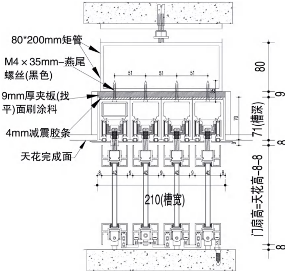
WP-A系列 宽盖四轨3+1联动门 四轨4+0联动门
