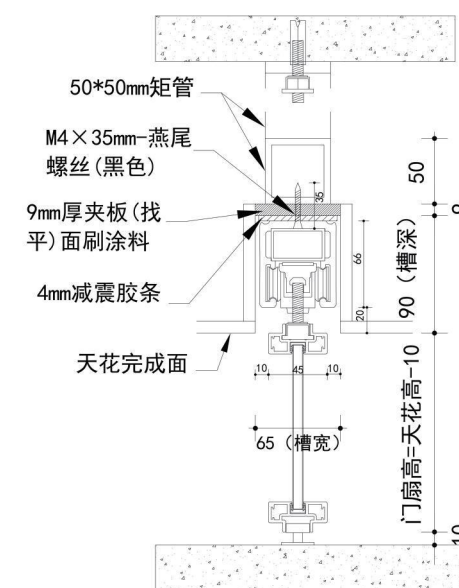
AP系列 单轨单开门 单轨反向同步门 单轨口袋门
