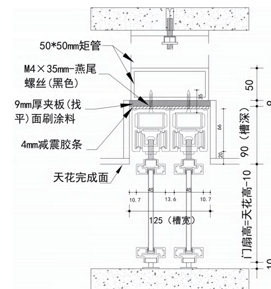
AP系列 双轨单开/双开门 双轨反向同步门
