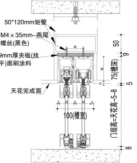
WM-B系列 窄盖双轨单开/双轨开门 双轨反向同步门 双轨2+0联动门
