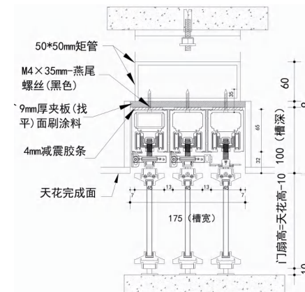
UP系列 三轨2+1联动门 三轨3+0联动门
