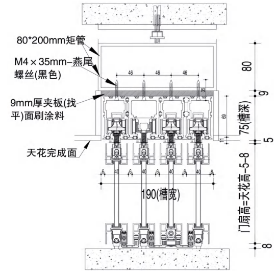
WM-B系列 窄盖四轨3+1联动门 四轨4+0联动门
