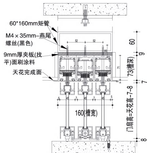
QM45-B装饰盖34mm-直驱微缝 三轨2+1联动门 三轨3+0联动门
