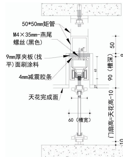
UP系列 单轨单开门 单轨反向同步门 单轨口袋门
