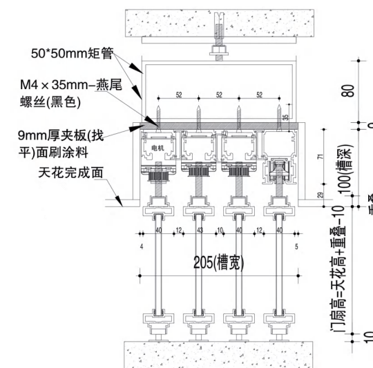
QM系列-40明装 三轨3+1联动门
