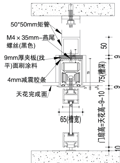
XP-A系列 宽盖单轨单开门 单轨反向同步门
