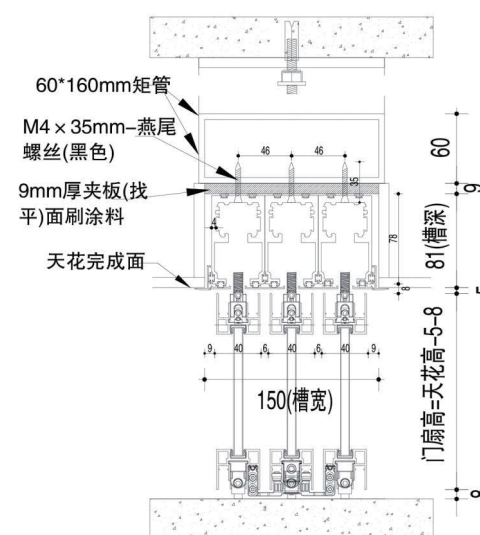
QM系列-40暗装 三轨2+1联动门 三轨3+0联动门
