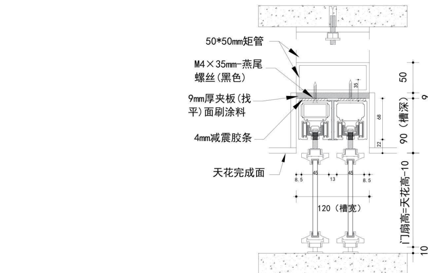
UP系列 双轨单开 双开门 双轨反向同步门
