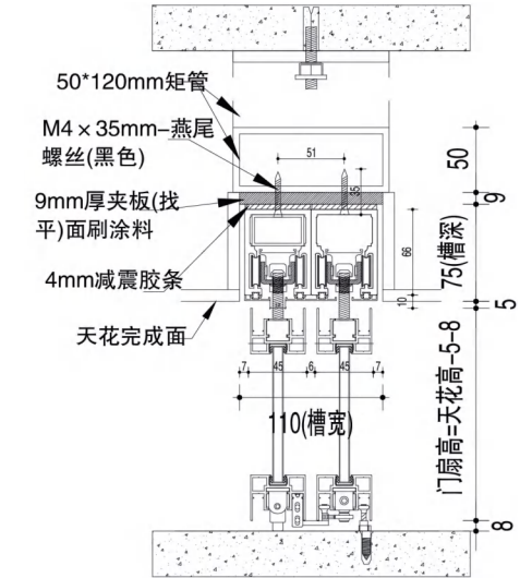
WP-B系列 窄盖双轨单开/双开门 双轨反向同步门 双轨2+0联动门
