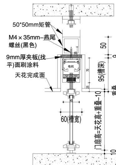
QM系列-45明装 单轨单开门 单轨反向同步门 单轨口袋门
