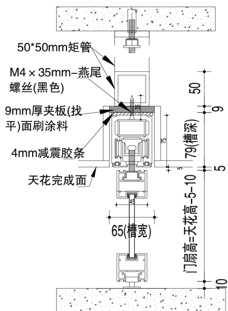
XP-B系列 窄盖单轨单开门 单轨反向同步门 单轨口袋门
