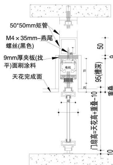
QM系列-40明装 单轨单开门 单轨反向同步门 单轨口袋门
