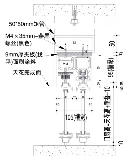
QM系列-40明装 双轨单开/双开门 双轨反向同步门
