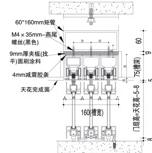
WP-B系列 宽盖三轨2+1联动门 三轨3+0联动门
