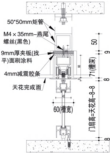
WP-A系列 窄盖单轨单开门 单轨反向同步门 单轨口袋门
