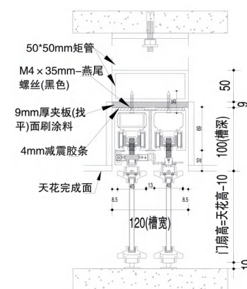
UP系列 双轨2+0联动门
