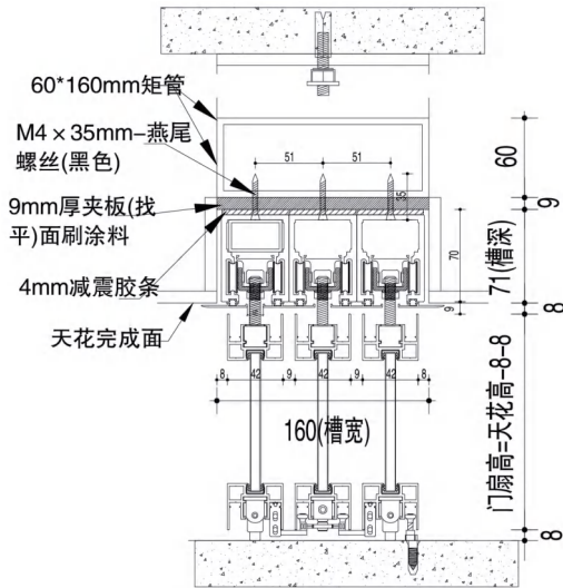
WP-A系列 宽盖三轨2+1联动门 三轨3+0联动门
