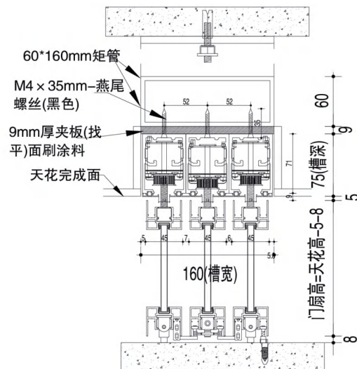
QM45-B装饰盖19mm-直驱微缝 三轨2+1联动门 三轨3+0联动门
