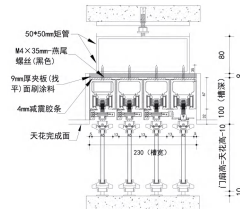
UP系列 四轨3+1联动门 四轨4+0联动门
