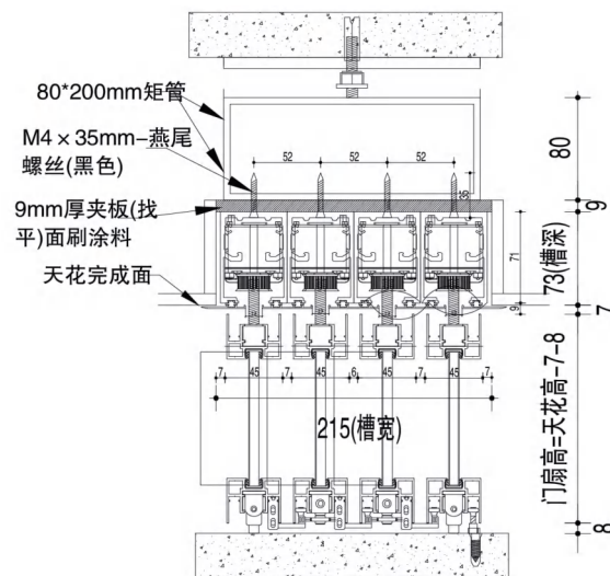
QM45-B装饰盖34mm-直驱微缝 四轨3+1联动门 四轨4+0联动门
