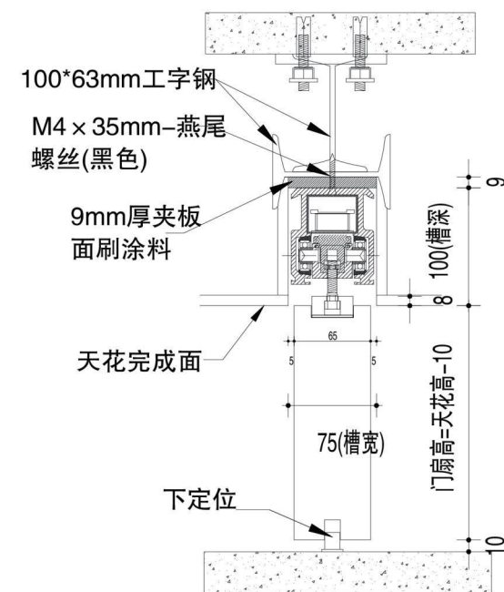
重型系列 单轨单开移门 单轨反向同步移门
