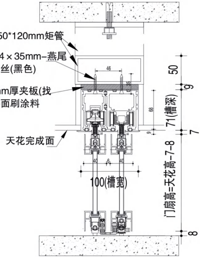
WM-A系列 宽盖双轨单开/双轨双开 双轨反向同步门 双轨2+0联动门
