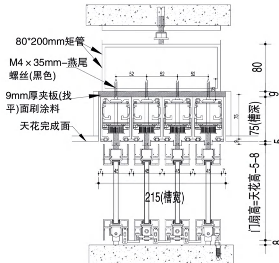
QM45-B装饰盖19mm-直驱微缝 四轨3+1联动门 四轨4+0联动门
