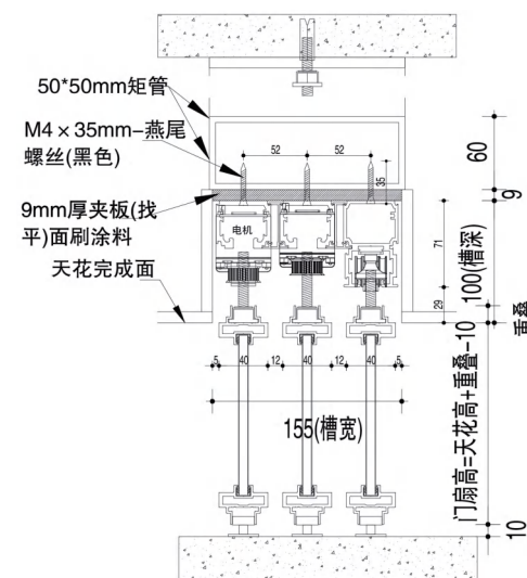
QM系列-40明装 三轨2+1联动门 三轨3+0联动门
