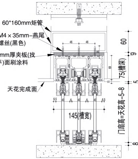
WM-B系列 窄盖三轨2+1联动门 三轨3+0联动门
