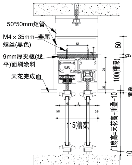
QM系列-45明装 双轨2+0联动门
