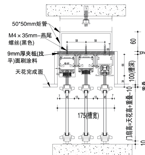
QM系列-45明装 三轨2+1联动门 三轨3+0联动门
