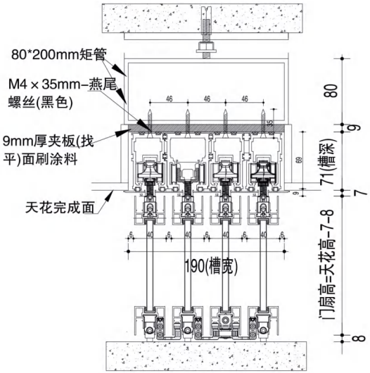
WM-A系列 宽盖四轨3+1联动门 四轨4+0联动门
