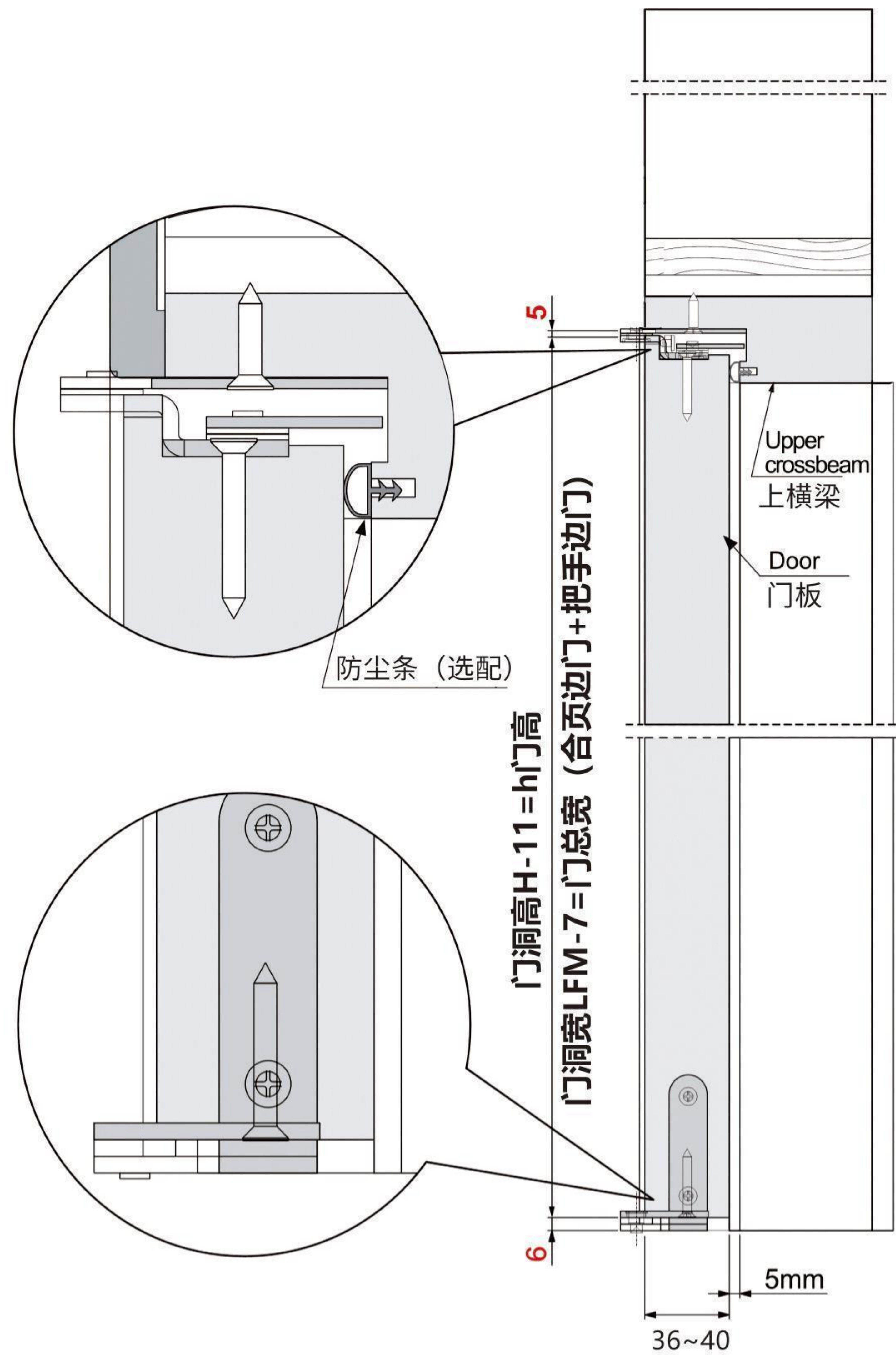
Vertical section (门框及门高参数图)
