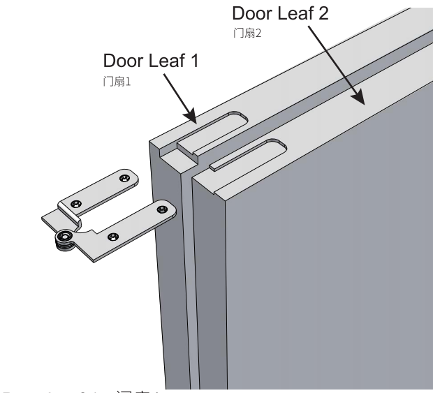
Door Leaf 1 / 门扇1
