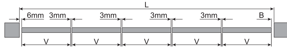
5 panels / 5扇门
