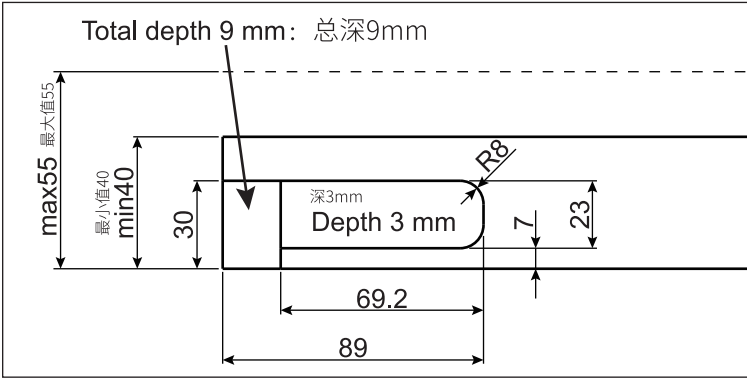
Door Leaf 1 / 门扇1
