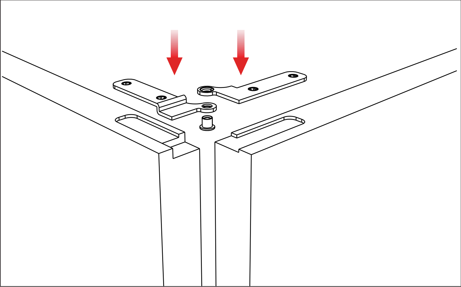
TOP HINGE / 顶部合页
