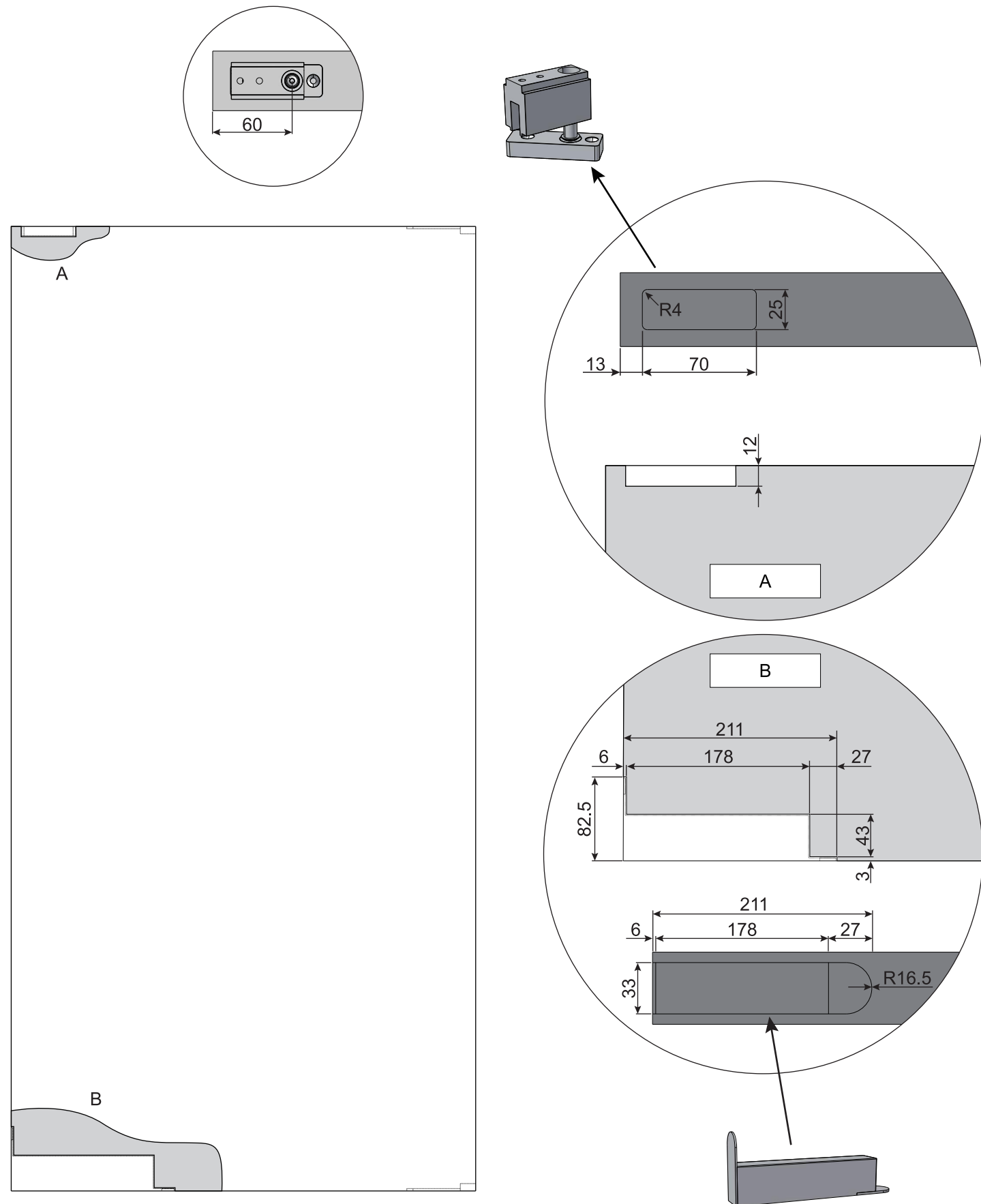
SECTION OF DOOR LEAF 1 / 第一扇门开孔图 (A)
