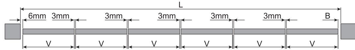
6 panels / 6扇门
