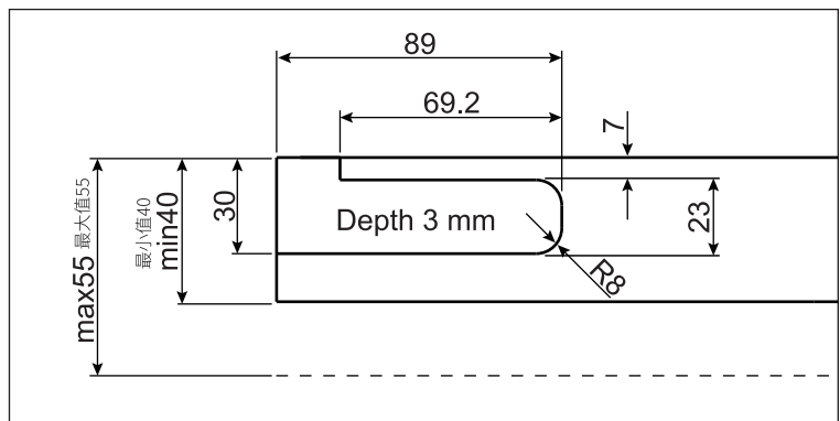
Door Leaf 2 / 门扇2
