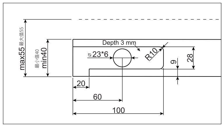
Door Leaf 3
