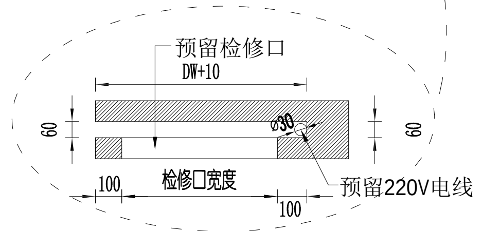
检修口尺寸图
