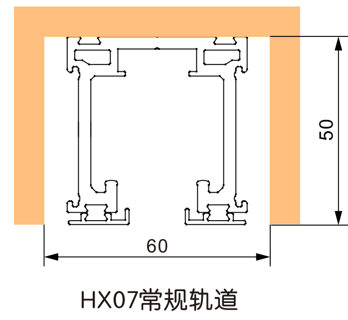
HX07常规轨道
