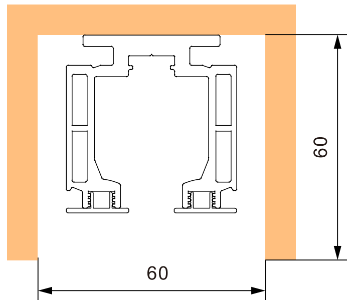
HX02常规轨道
