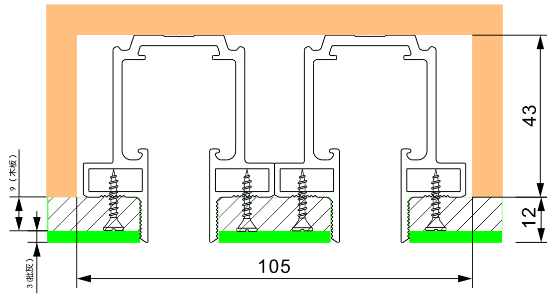
HX06线型双轨道
