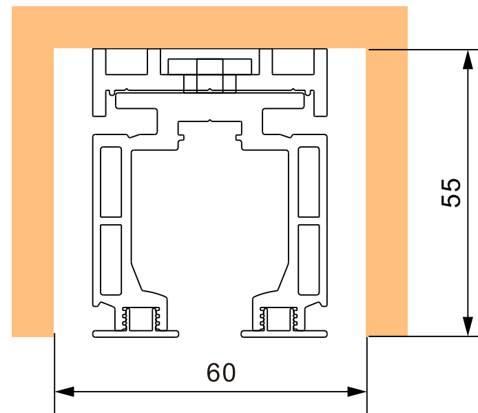
HX02免检修 (轨道+顶座)
