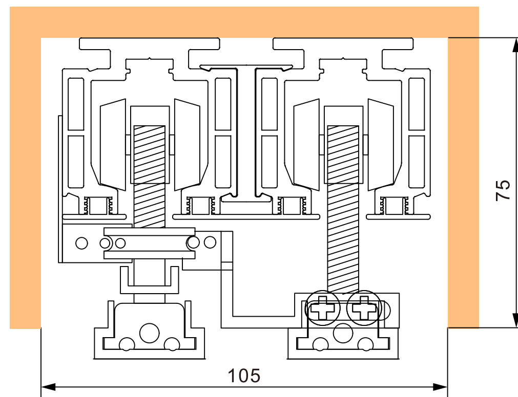
HX02双轨轨道/门上联动
