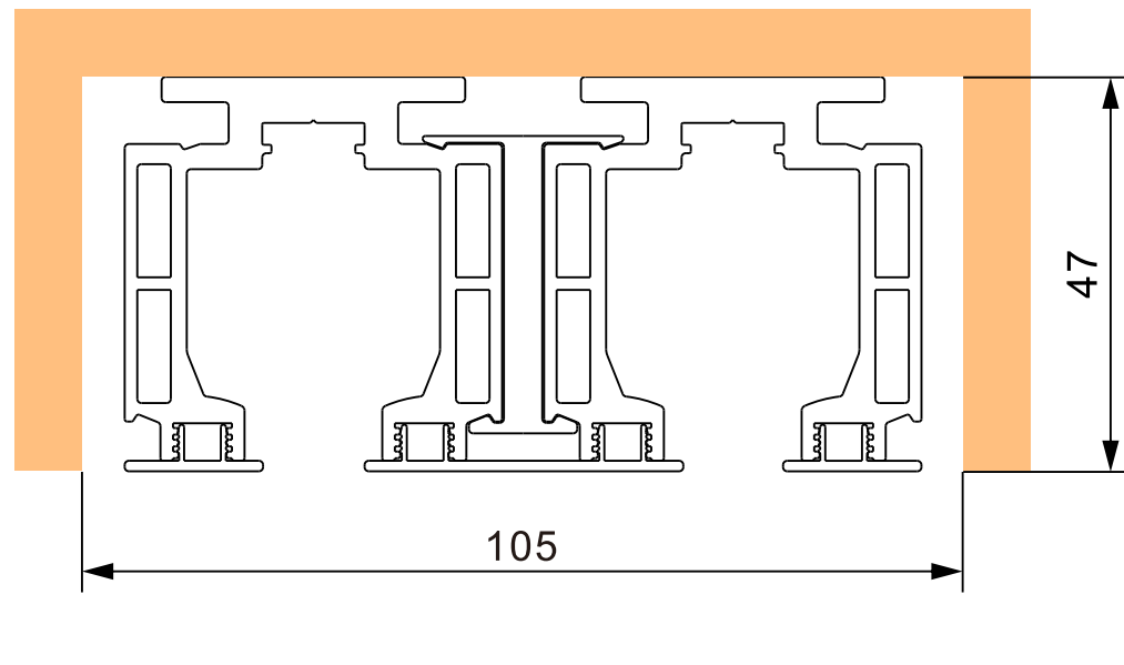
HX02双轨轨道/门下联动
