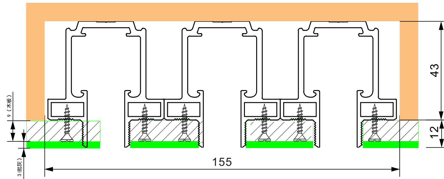
HX06线型三轨道
