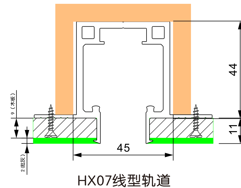
HX07线型轨道
