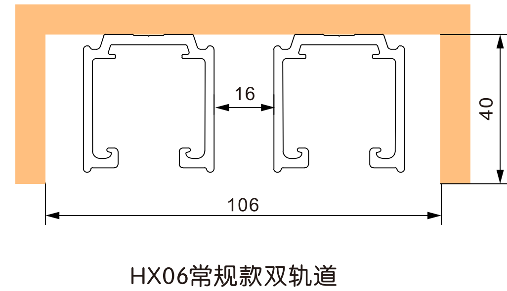
HX06常规款双轨道
