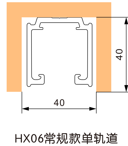
HX06常规款单轨道
