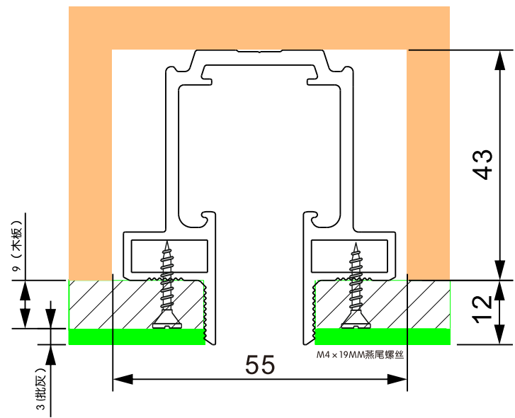
HX06线型单轨道
