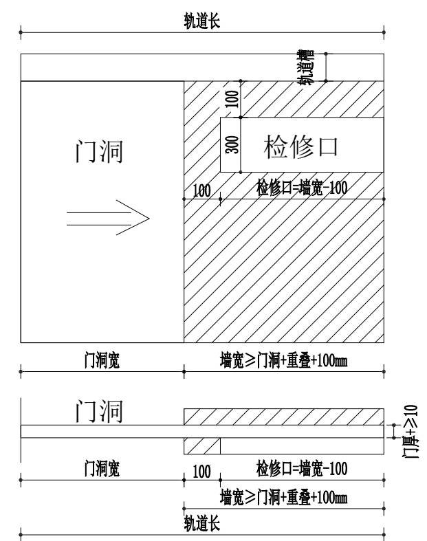
口袋门留检修口示意图
