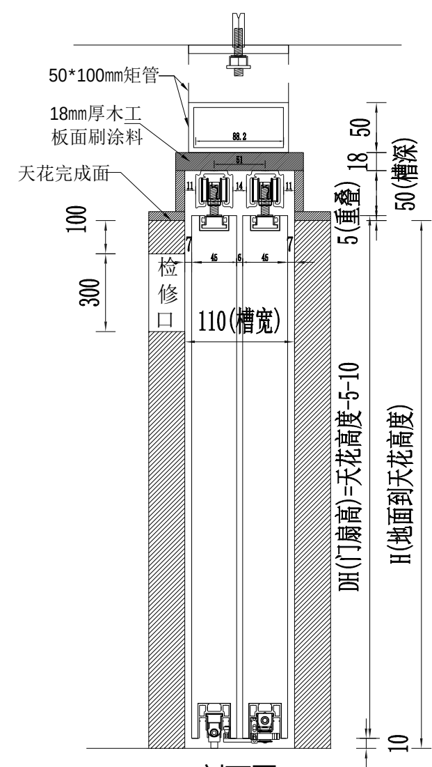
剖面图
