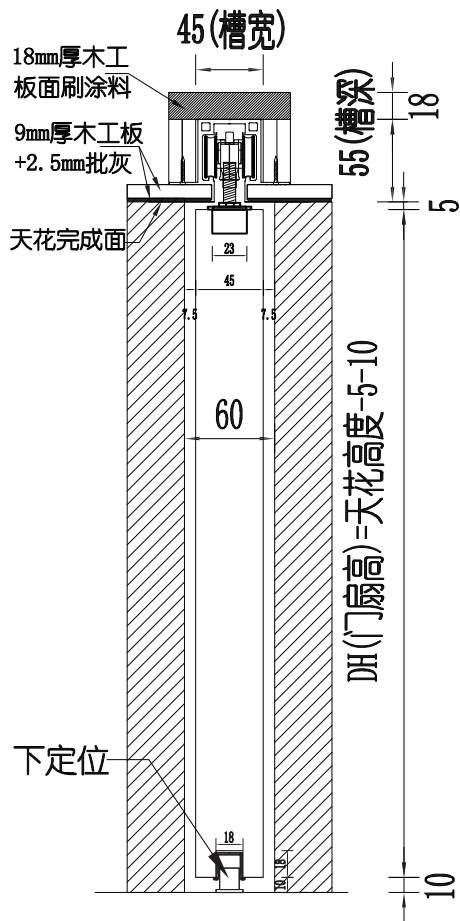
线性款剖面图
