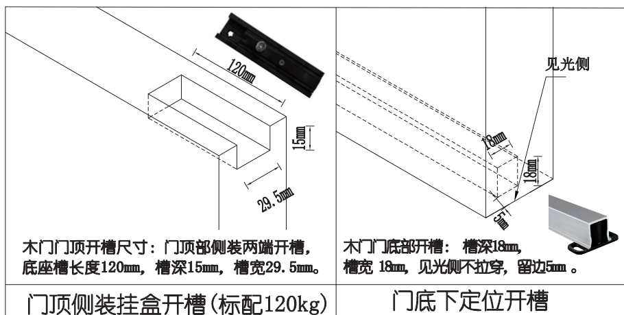
线性款剖面图
