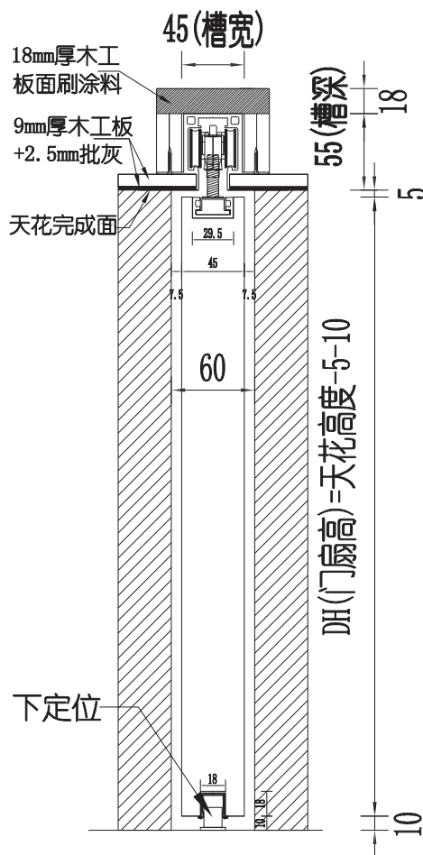
线性款剖面图
