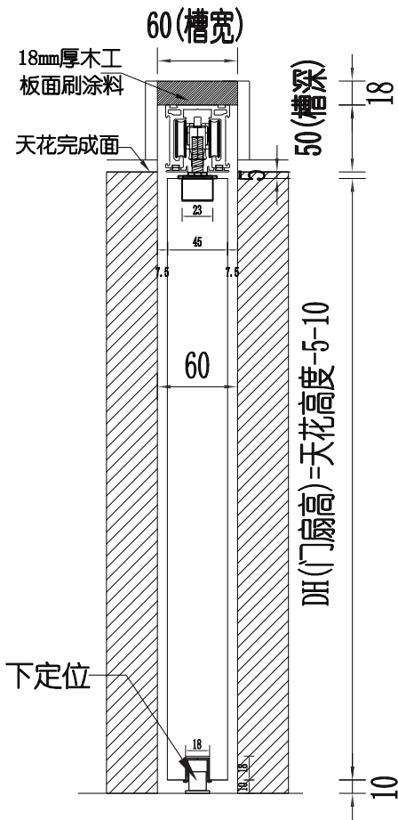
常规款剖面图
