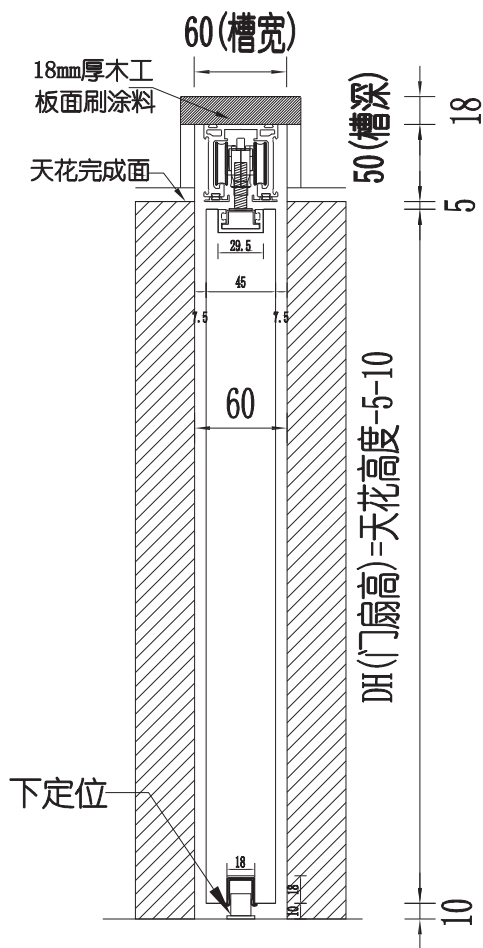
常规款剖面图
