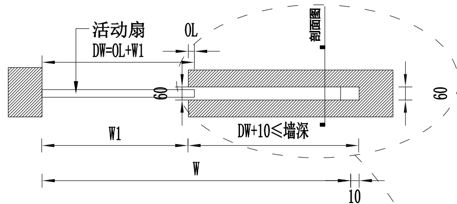
单轨口袋门
